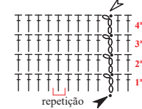
Diagrama 3 - Bico de acabamento (B)
