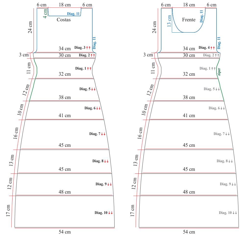
Esquema de medidas
