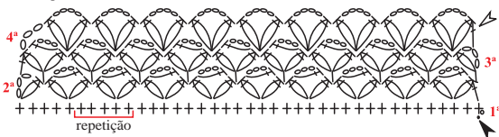
Diagrama 6 - ponto fantasia (D)
