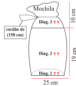
Esquema de medidas Parte de trás = Parte da frente
